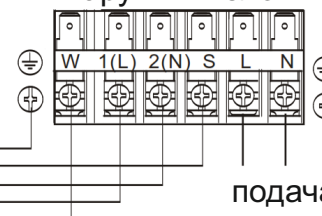
наружный блок
