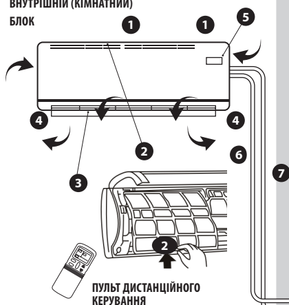
Стрілками відображено напрямки руху повітря
